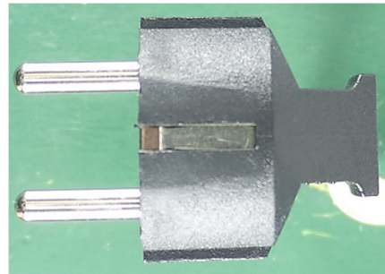
Verwendeter Biegeschutz A(schmäler)/ bend prevention A(small)
